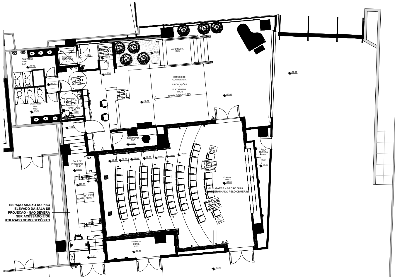
01 PL. BAIXA - TÉRREO (TORRE 2) Escala: 1/100
